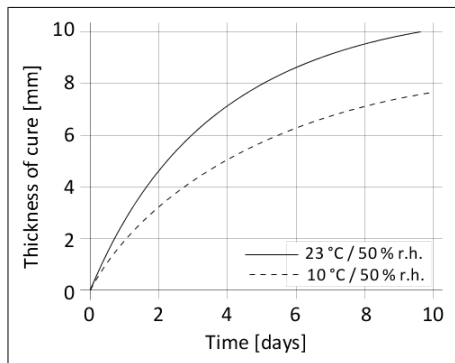
1. diagram: A Sikaflex®-515 térhálósodási sebessége
