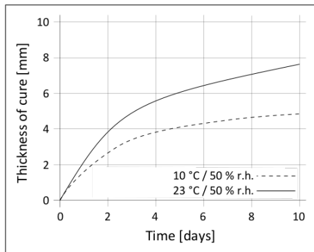
1. diagram: A Sikaflex®-529 Evolution térháló-sodási sebessége
