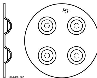
Sarnafast RT 82x40 alátéttárcsa
