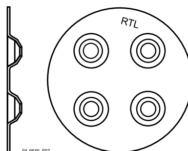
Sarnafast RTL 82x40 alátéttárcsa
