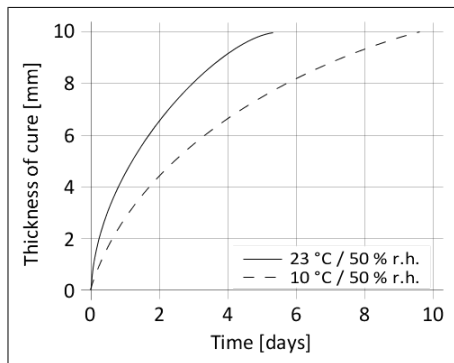
1. diagram: Sikaflex®-298 FC kötési sebessége
