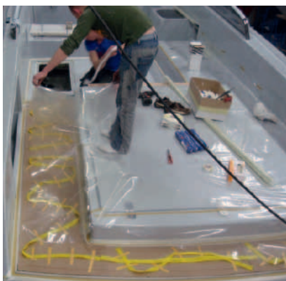
Fig. 15 Vacuum press
