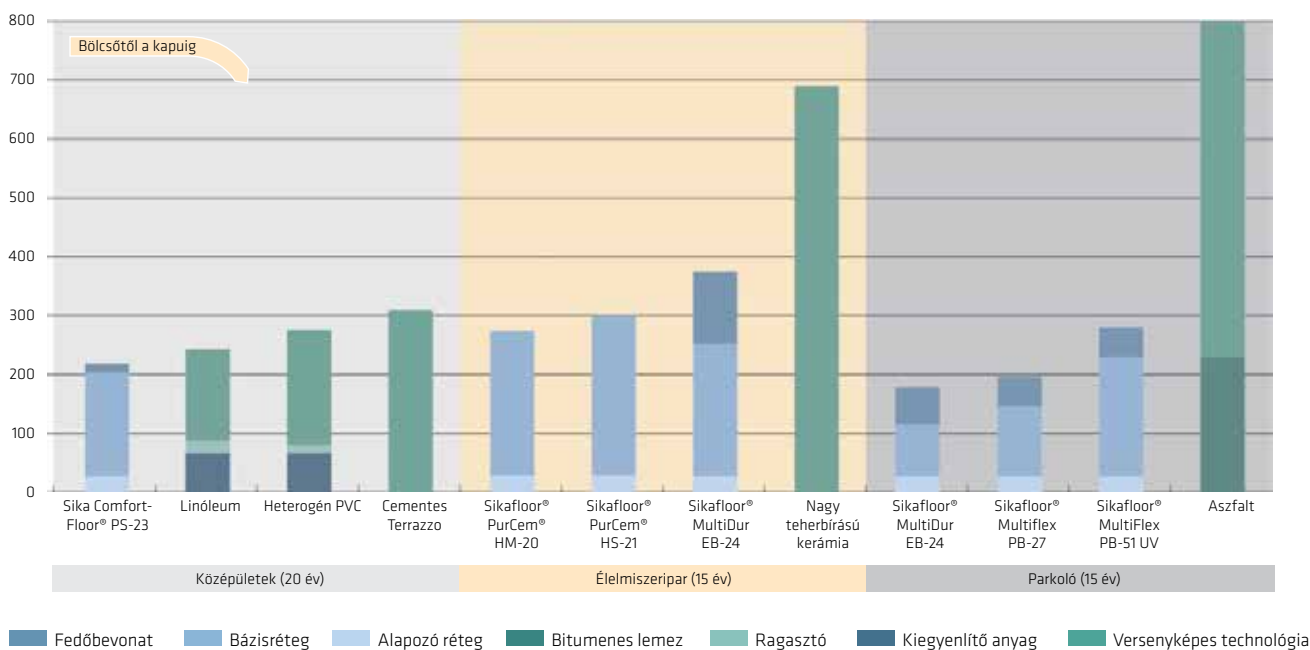
1 m 2 -nyi padlóburkolat kumulatív energiaigénye [MJ/m 2 ]
