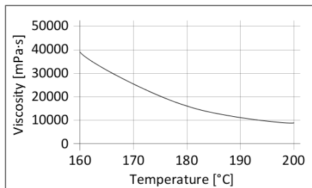
1. diagram: Viszkózitás a hőmérséklet függvényében
